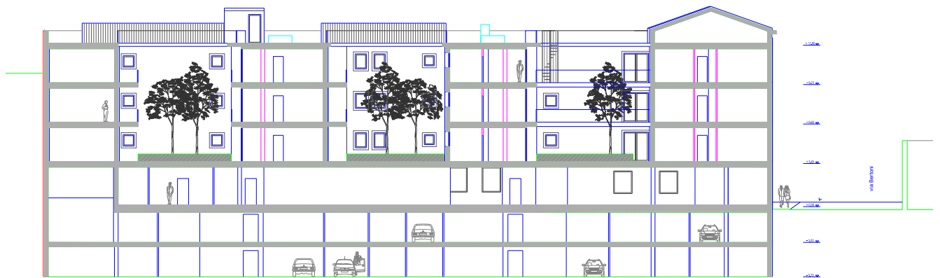
Sezione
