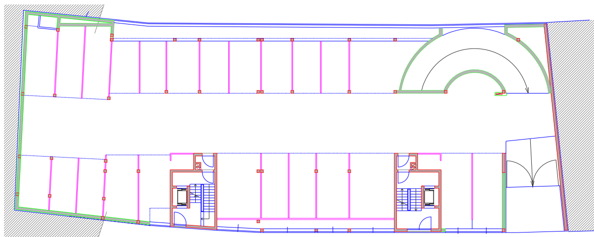
Planimetria Interrato -1
